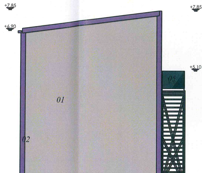
FATADA POSTERIOARA - VEST
