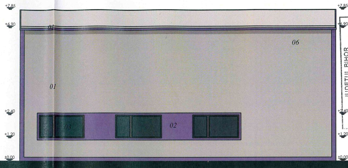
FATADA LATERALA DREAPTA - NORD
